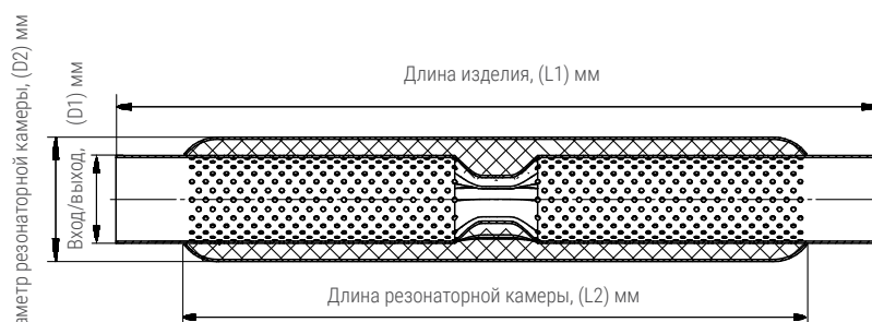
Чертёж стронгера универсального с формованным диффузором
