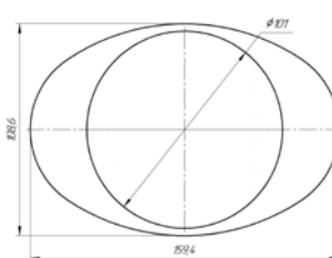
Чертёж переходника пламегасителя с размерами
