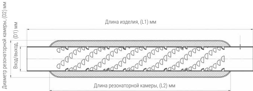
Чертёж стронгера универсального с жаброобразным внутренним узлом
